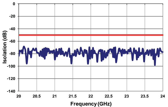
Isolation (20-24 GHz)
