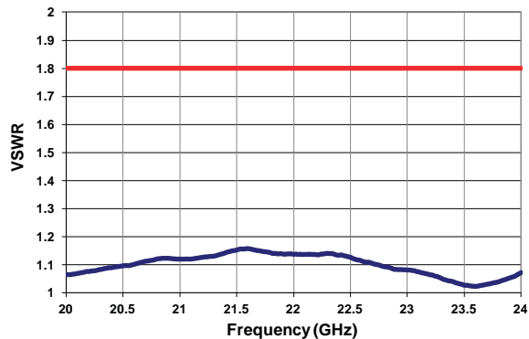
VSWR ( 20-24 GHz )
