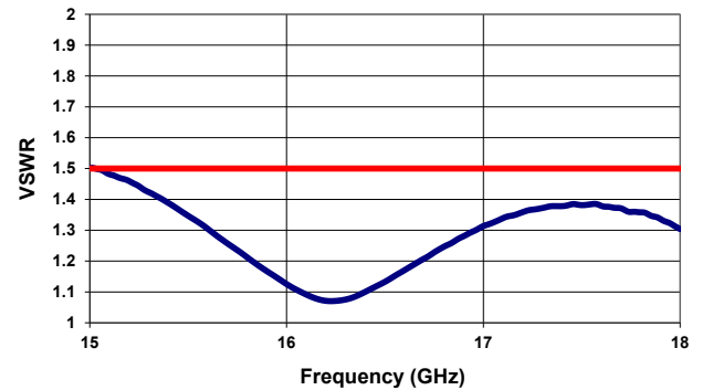
VSWR ( 15-18 GHz )
