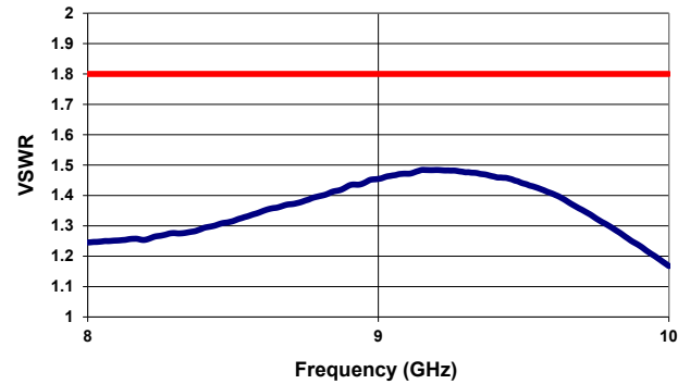
VSWR ( 8-10 GHz )
