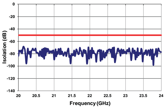
Isolation (20-24 GHz)
