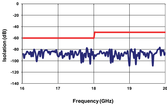
Isolation (16-20 GHz)
