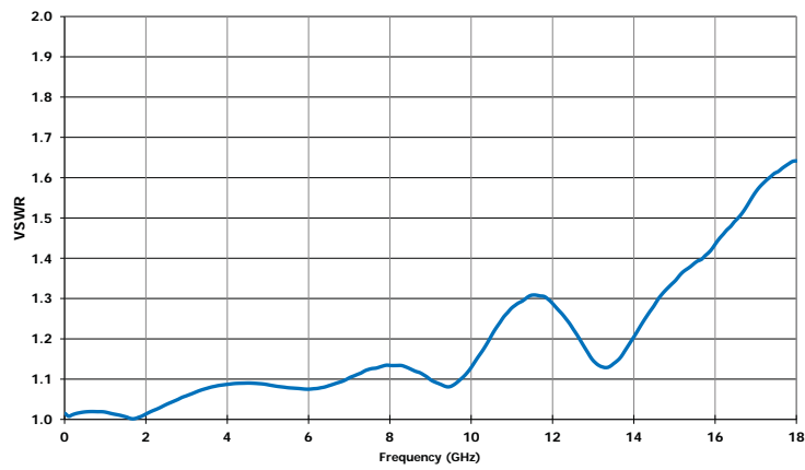
VSWR (DC - 18GHz)
