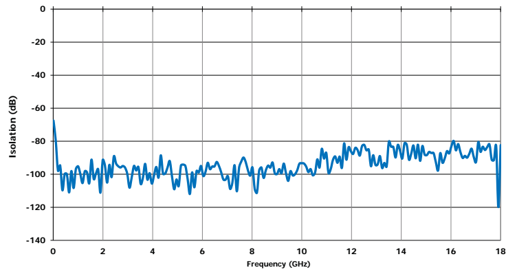
Isolation (DC - 18GHz)
